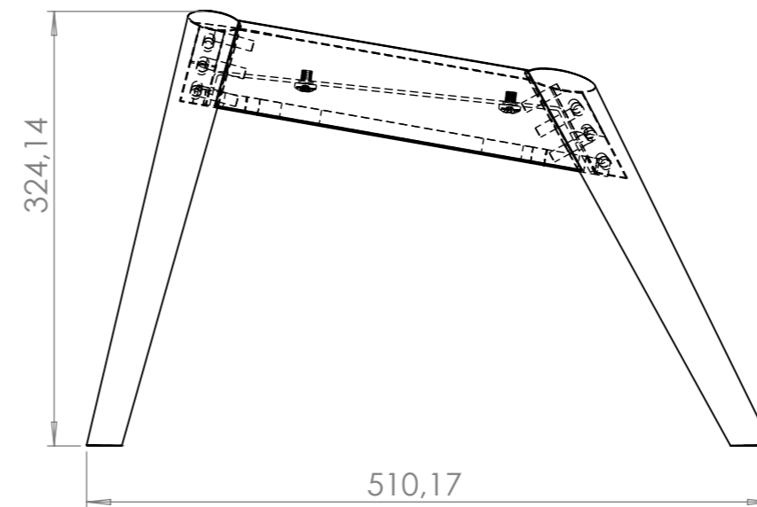
SIZE treunderstell innledende tegning for mockup
